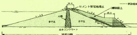
決定された多摩湖の堤防強化工法
