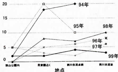
北川の水質推移(COD mg/l)
